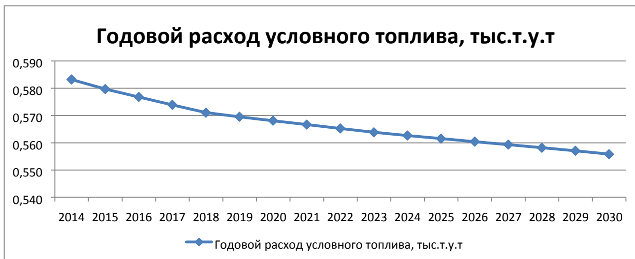
Рис. 6. Перспективный баланс по твердому топливу
