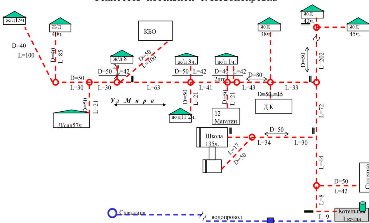
Теплосеть котельной с. Новопокровка
